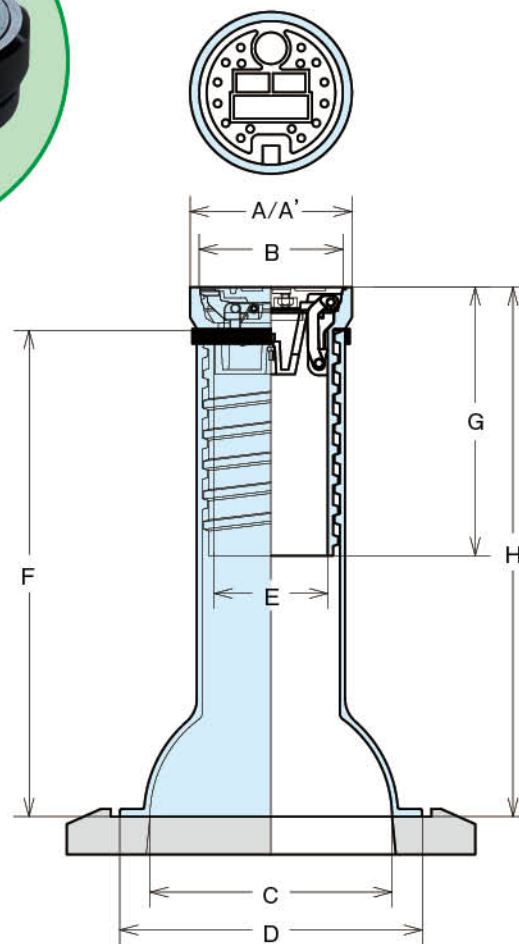
除雪対応型
